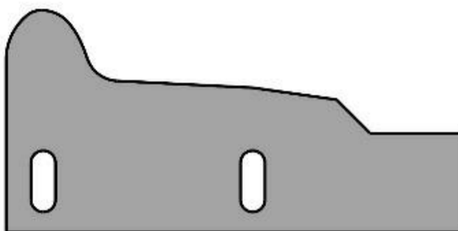
Копир для станка PT905, UBB112 PG
